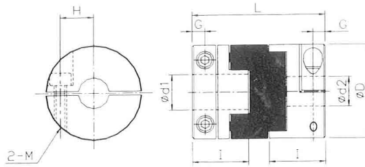
外徑 \varnothing D40 \sim \varnothing D63
